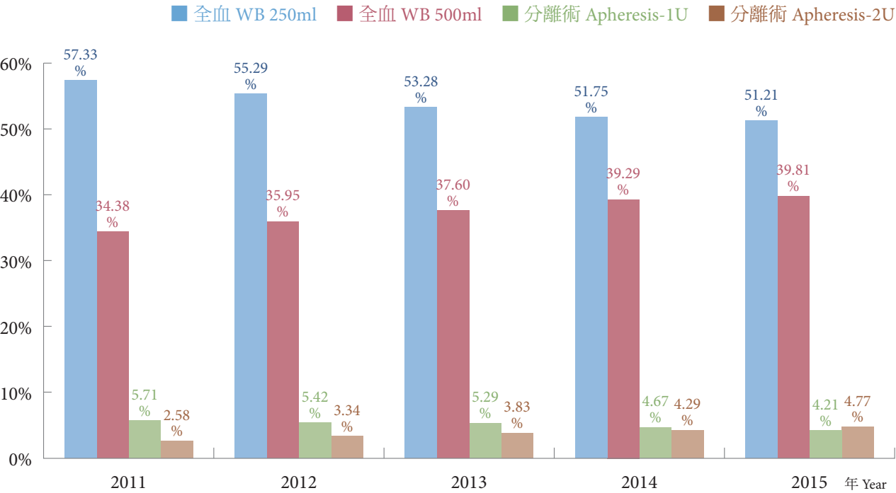
近五年捐血類型分析 Types of Blood Donation, 2011-2015
