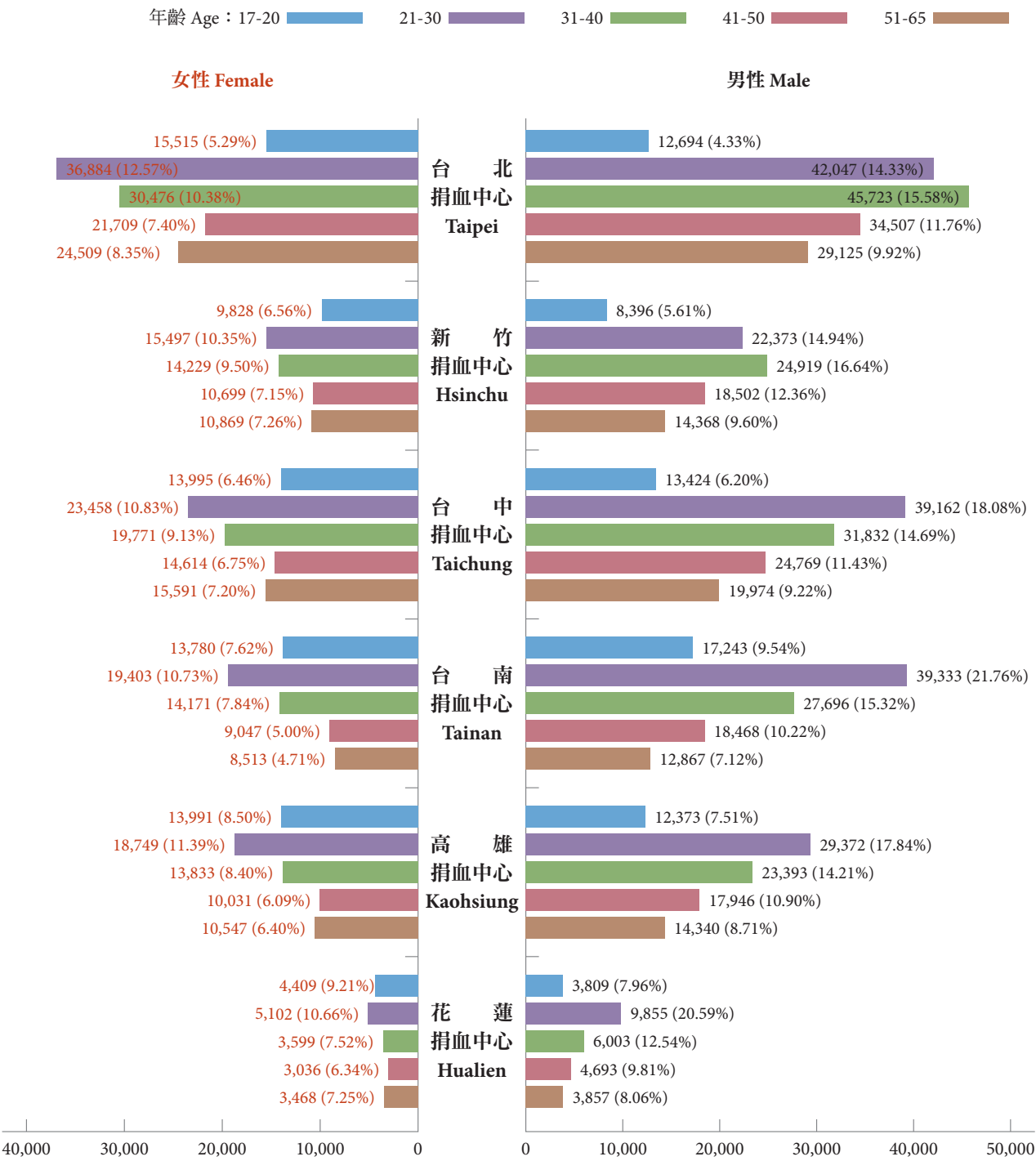
104年捐血年齡及性別分析—依人數 Distribution of Blood Donor by Gender and Age in 2015
