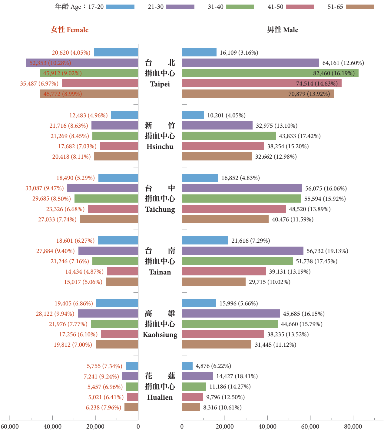
104年捐血年齡及性別分析—依人次 Distribution of Blood Donation by Gender and Age in 2015
